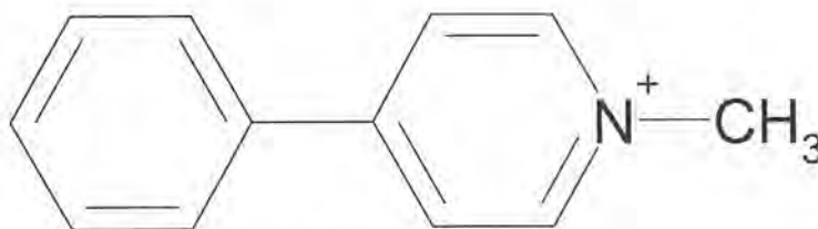
MPP +
