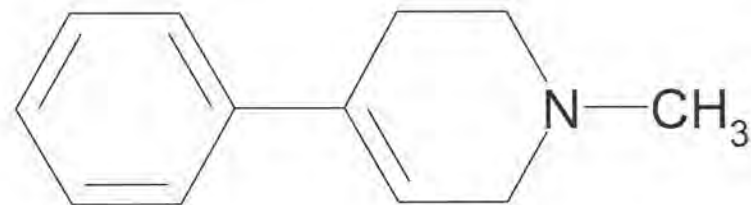
MPTP
